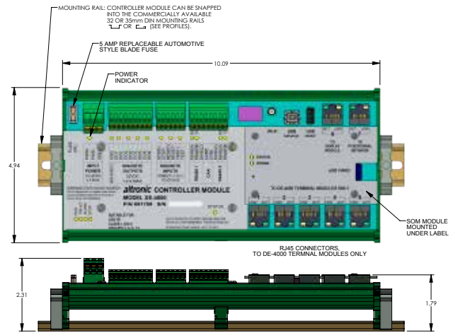
CONTROLLER MODULE
